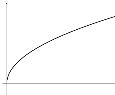
(b) y = \sqrt{x}
