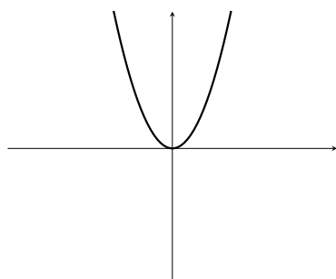
(d) y = x^2
