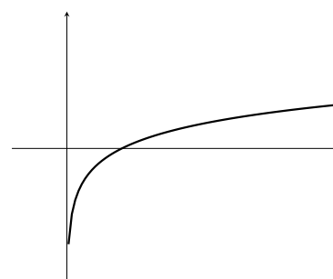
(f) y = \ln x
